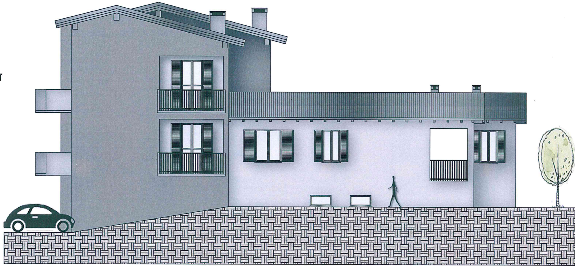
PROSPETTO OVEST
