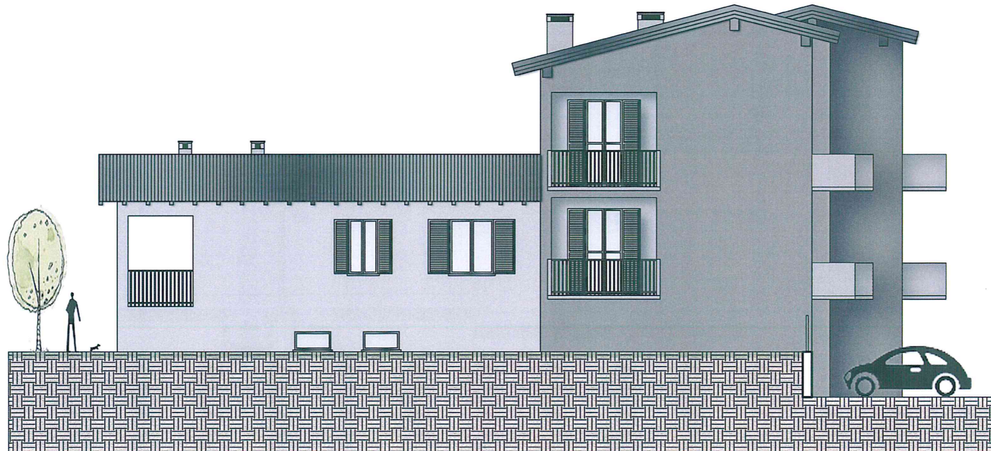
PROSPETTO EST
