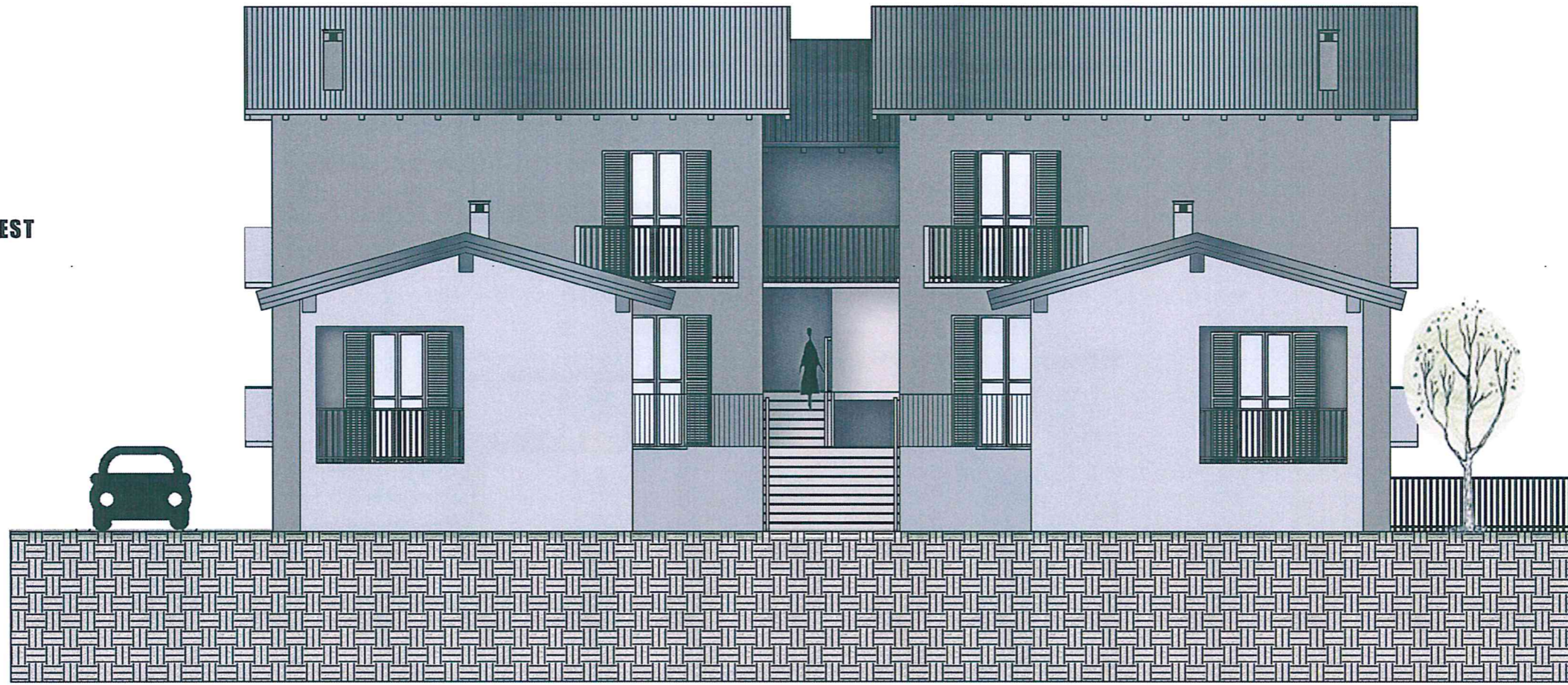
PROSPETTO SUD
